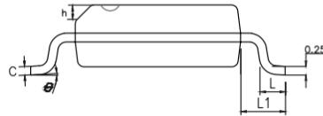
SSOP-10L
