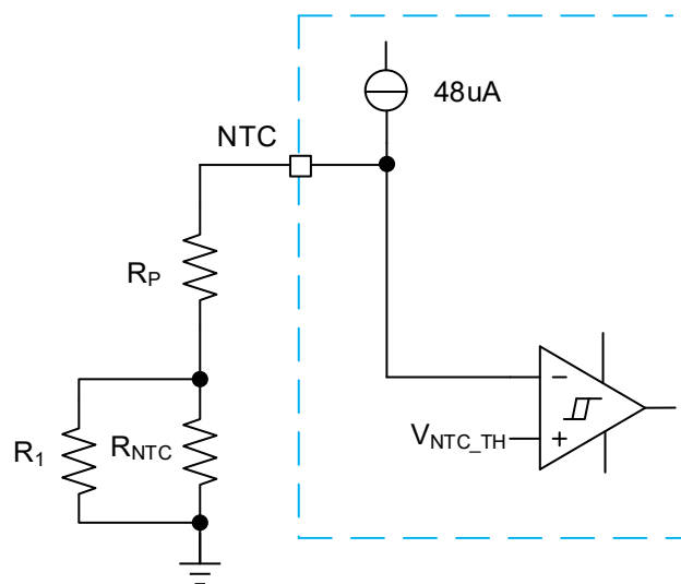
Fig. 5. NTC Protection
