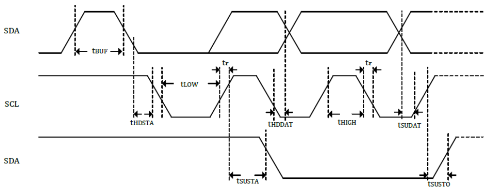
I2C协议
