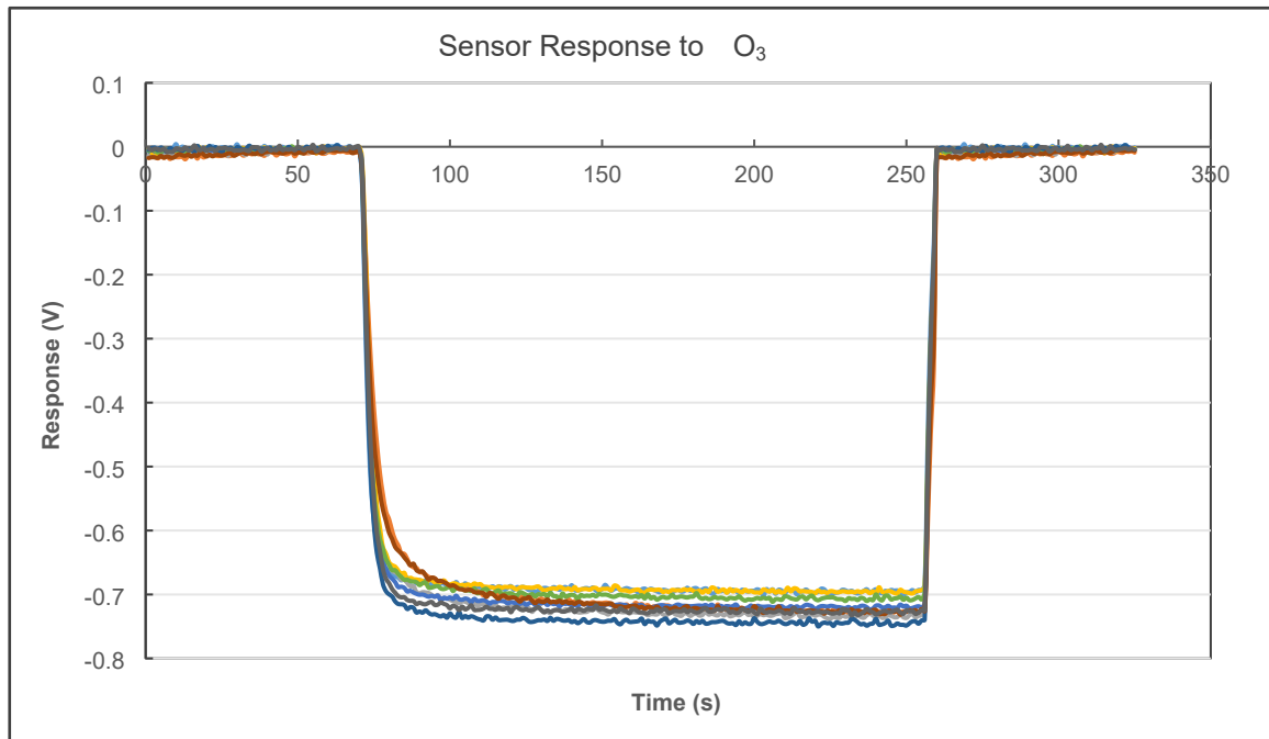
臭氧传感器基线的响应恢复曲线
