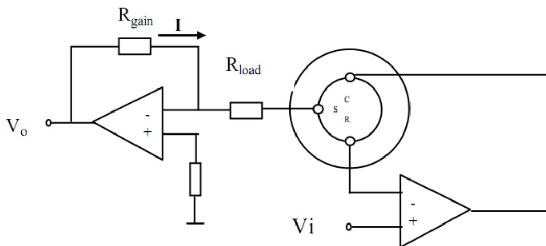
臭氧传感器的基本测试电路。
