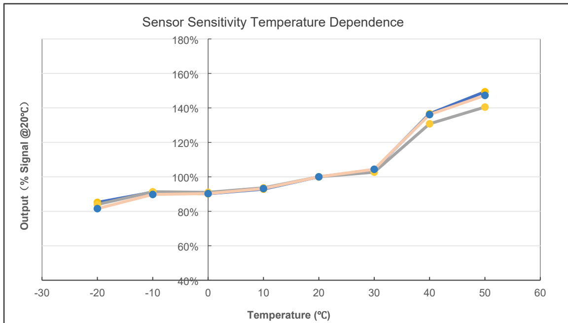
臭氧传感器灵敏度的温度依赖性曲线
