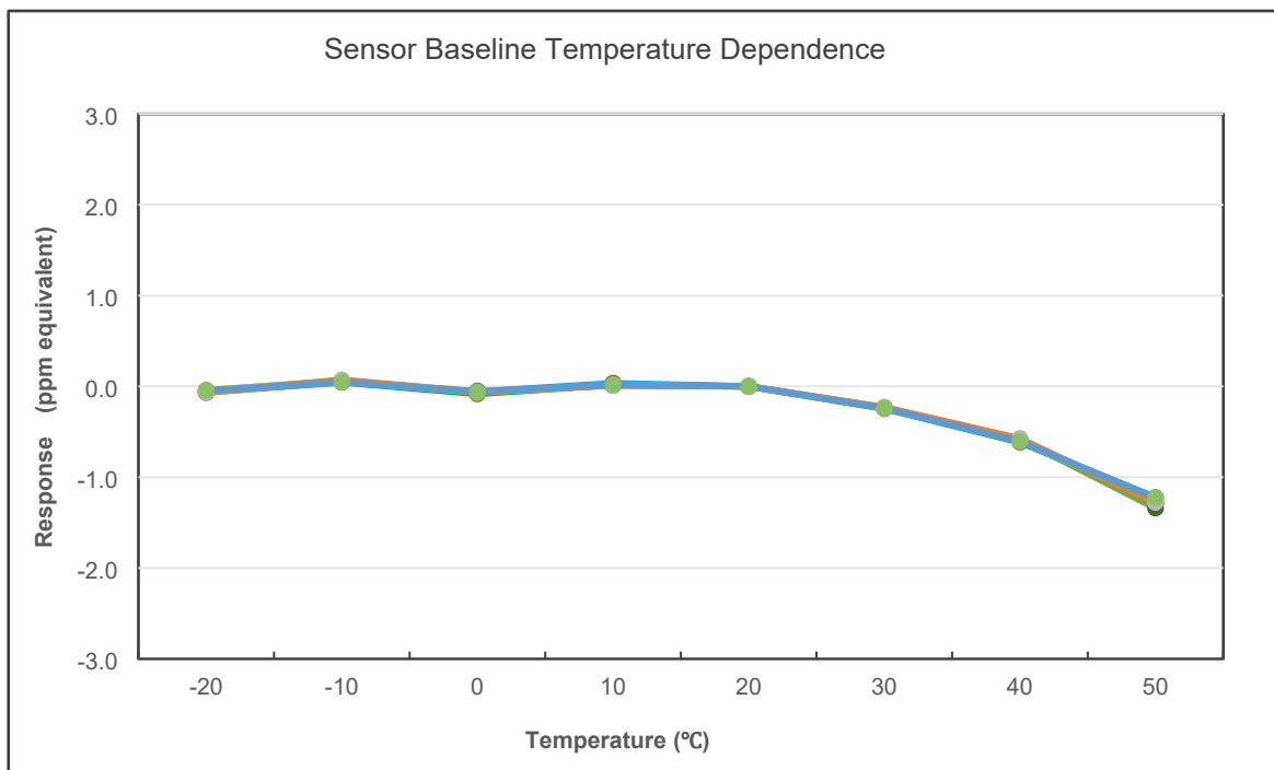
臭氧传感器基线的温度依赖性曲线
