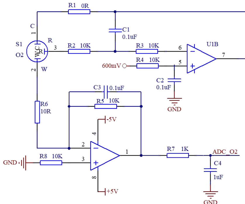
MS-O2-29BMEUL无铅氧气传感器的推荐电路
