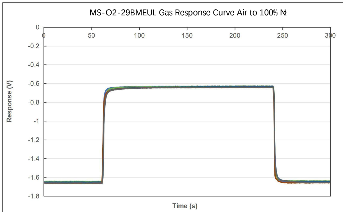
MS-O2-29BMEUL无铅氧气传感器响应恢复曲线
