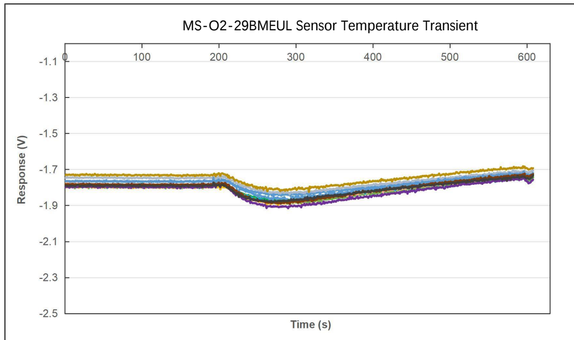
MS-O2-29BMEUL 氧气传感器不同温度下瞬变的信号恢复曲线
