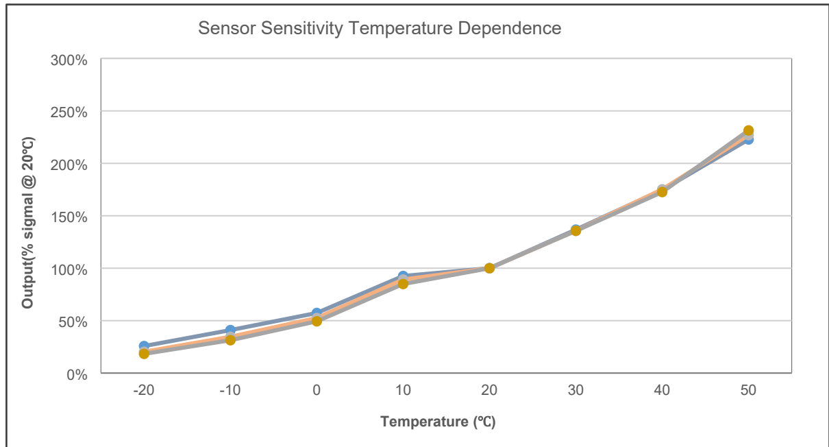
氢气传感器传感器灵敏度的温度依赖性曲线
