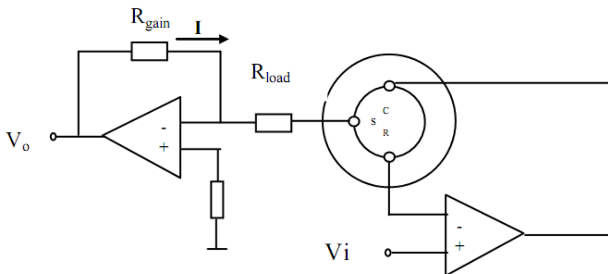
氢气传感器的基本测试电路
