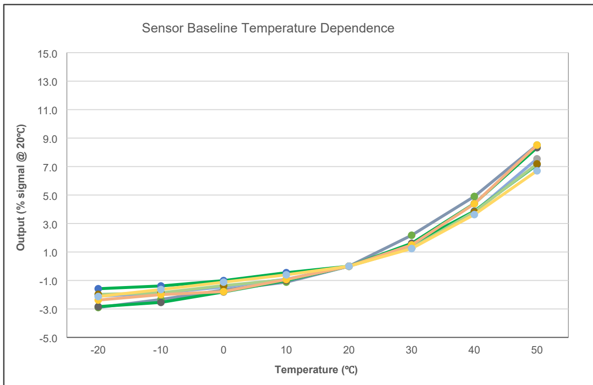
氢气传感器传感器基线的温度依赖性曲线
