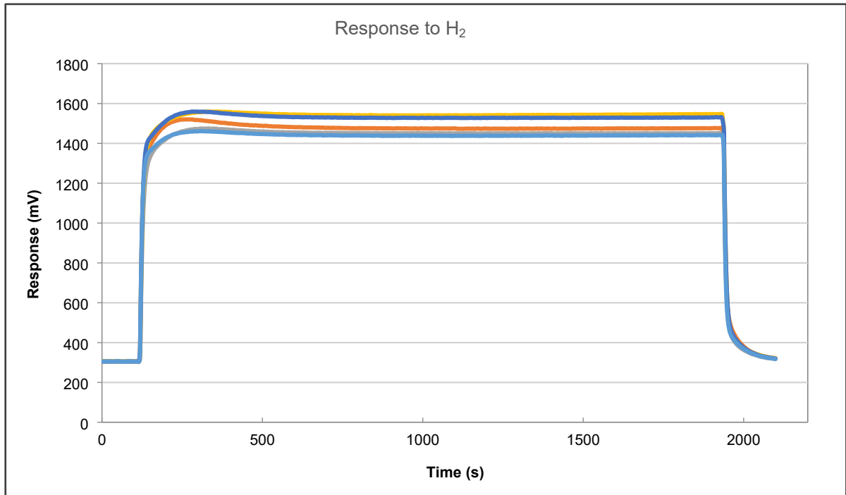
氢气传感器响应恢复曲线
