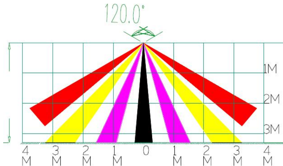
吸顶视图
