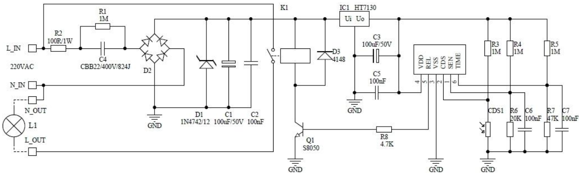
MS-DP-36BPF数字热释电传感器典型参考电路
