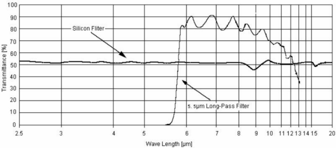
滤光片光谱图
