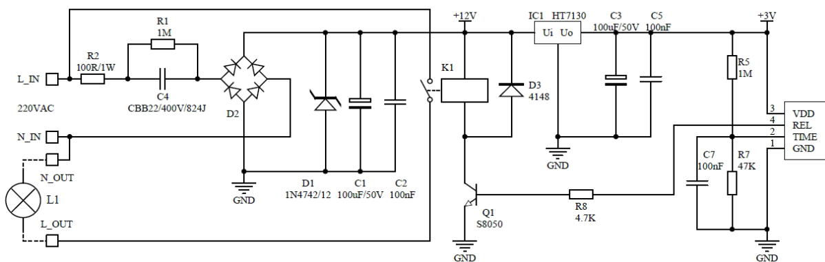
MS-DP-36BP4数字热释电典型应用电路
