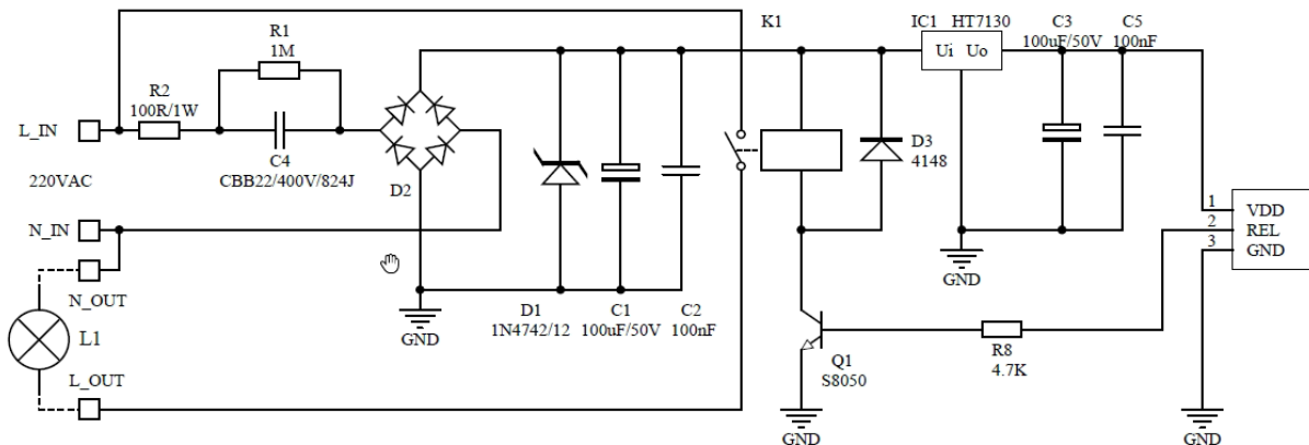
MS-DP-36BP3数字热释电典型应用电路
