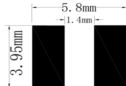
电路板布线图 (公差 \pm 0.2mm)
