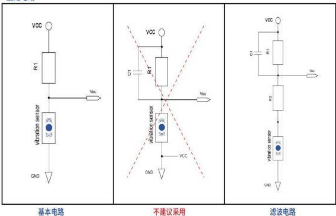
应用电路
